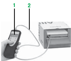
Конфигурирование ПЧ в упаковке с помощью мультизагрузчика WV3 A8 121+ кабель WV3 A8 126
