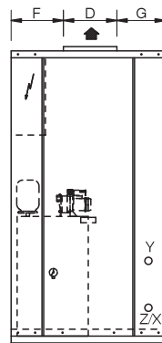
Вид "А-А"
