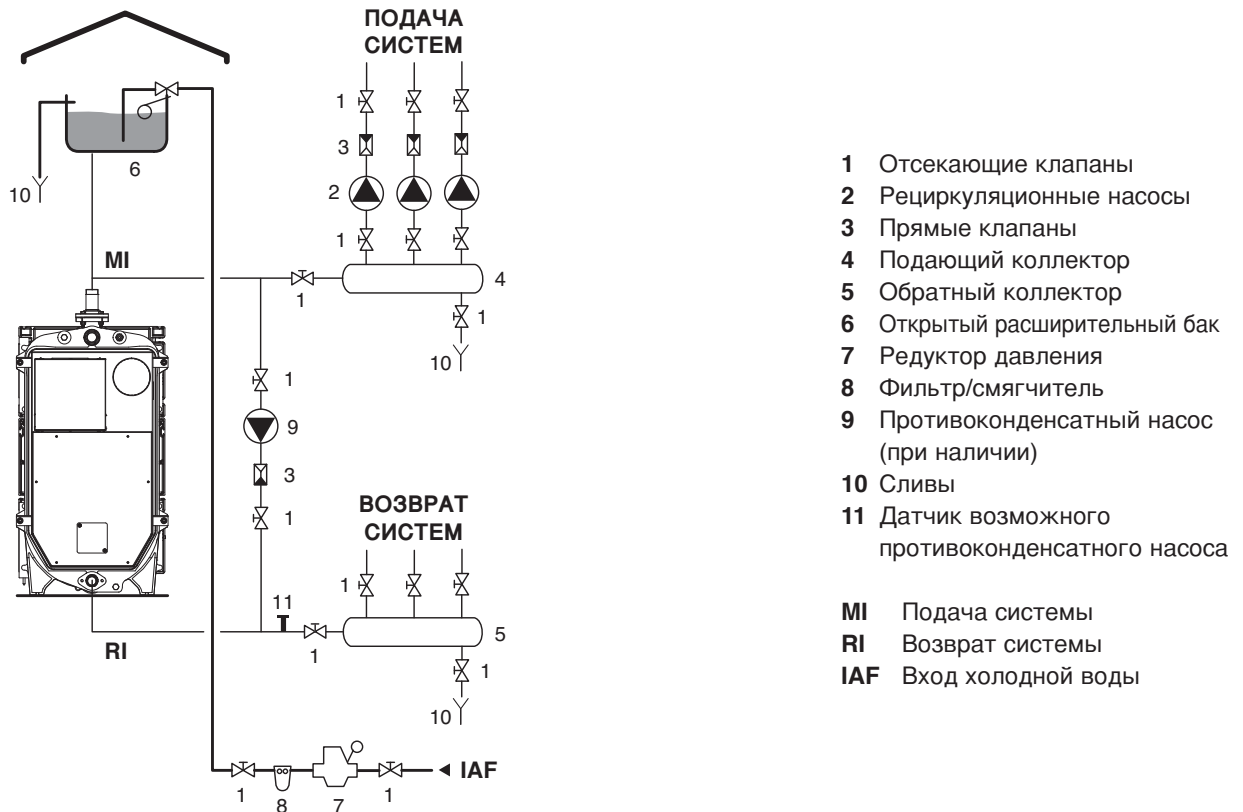
Схема 1: котел PIROWOOD, непосредственно соединенный с системами
