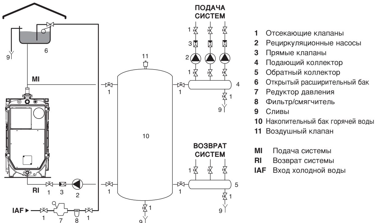
Схема 2: котел PIROWOOD с накопительным баком горячей воды для питания систем
