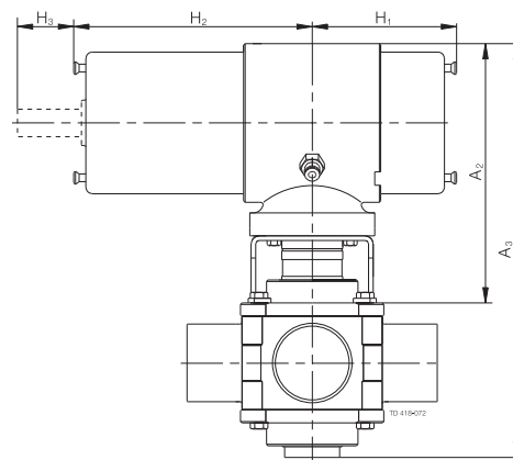
б. МН53 с пневмоприводом типа КН631
