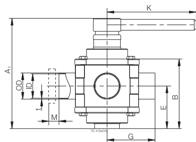
а. МН53 с ручкой Рис. 1. Размеры
