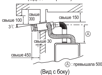
Расположение дымохода относительно стен и потолка. (Един измер. мм)
