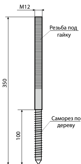
Универсальный анкер
