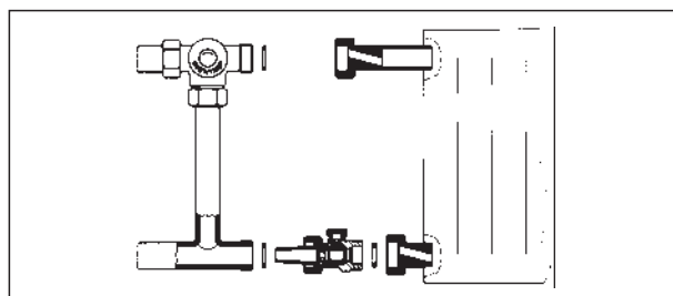
Конусная втулка с запорным устройством и сгоном:
