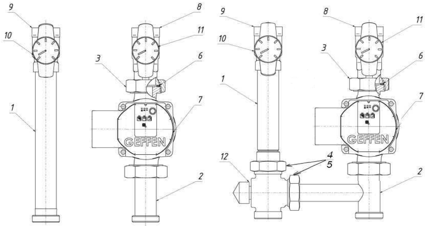
Модуль прямой
