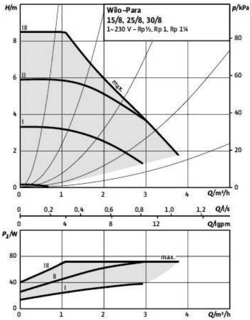
Др-в (переменный)
