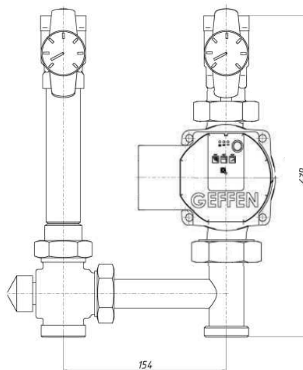
Модуль смесительный
