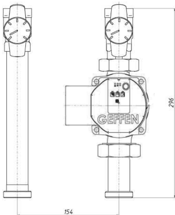
Модуль прямой
