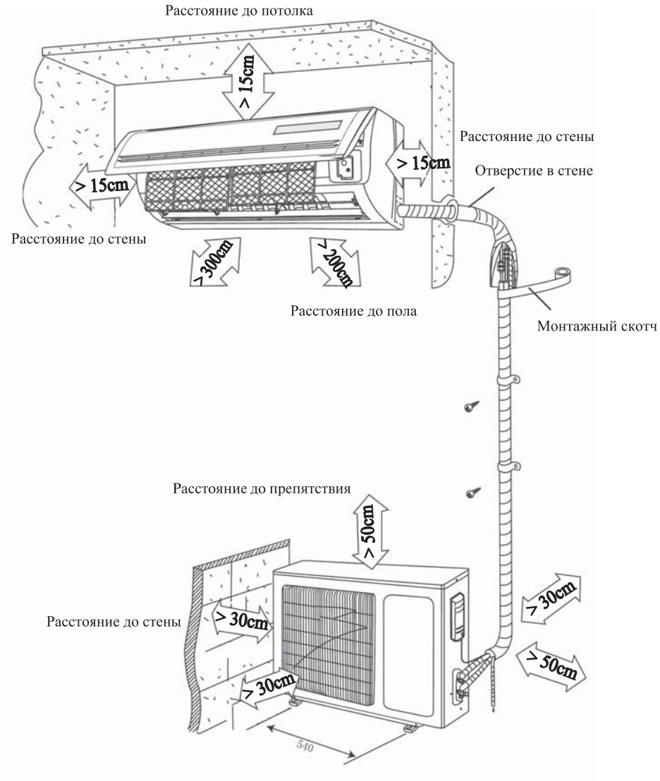
Рис. 8.1 Требования по размещению блоков
