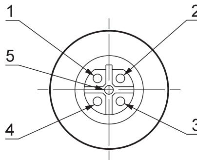
Рис. 1 Разъём M12, IP 65
