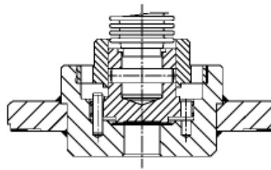
Разгрузочная головка для типоразмеров, начиная с DN 125
