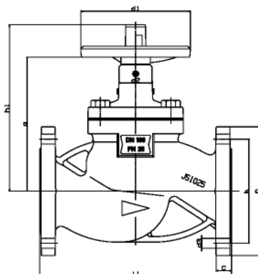
a и d2 размеры с изоляцией
