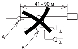
Рисунок 1. Не более двух разветвителей в магистральной трубе
