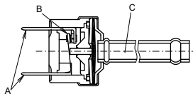
Схема реле высокого давления
