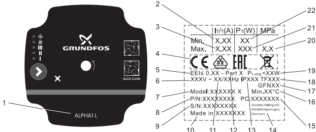
Նկար 1 ALPHA1 L պոմպի ֆիրմային վահանակ
