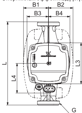
17-сүр. Тыш өлчөмдөрү
