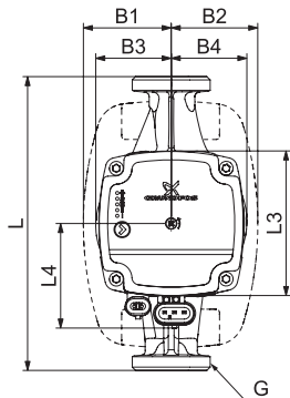
19-сүр. Тыш өлчөмдөрү
