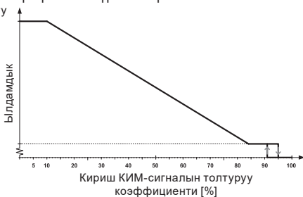
14-сүр. ALPHA1 Lги КИМ-сигналды башкаруучунун профили
