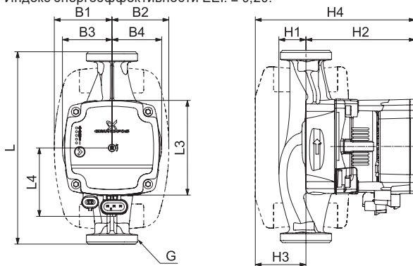
Рис. 17 Габаритные размеры
