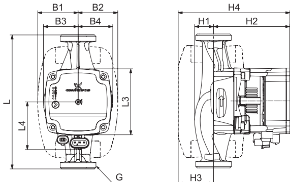
Նկար 19 Գաբարիտային չափսեր
