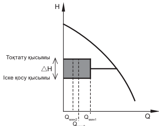
50-сур. Іске қосу және тоқтату қысымы ( \Delta H ) және минималды шығын мәндері арасындағы айырмашылық
