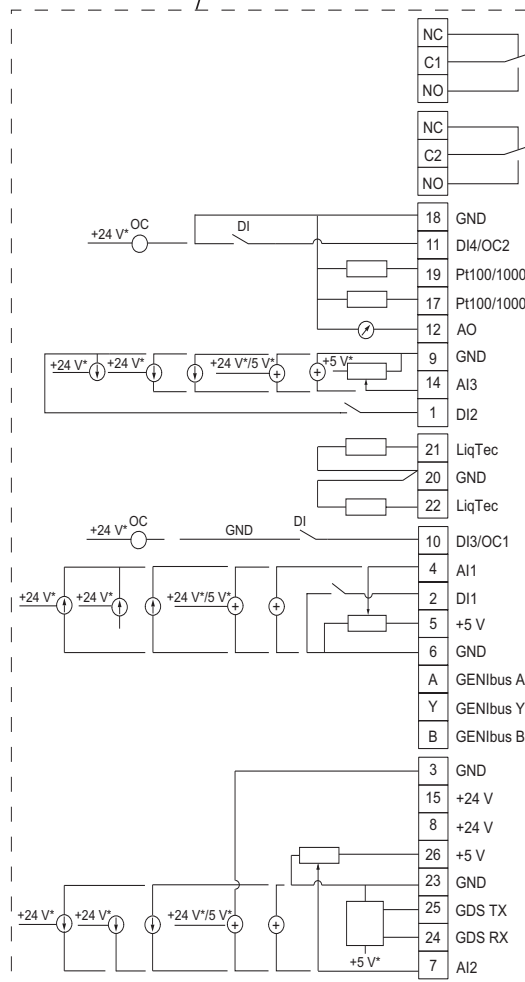
Рис. 8 Клеммы соединений, насосы CRE, CRIE, CRNE, CRTE и MTRE
