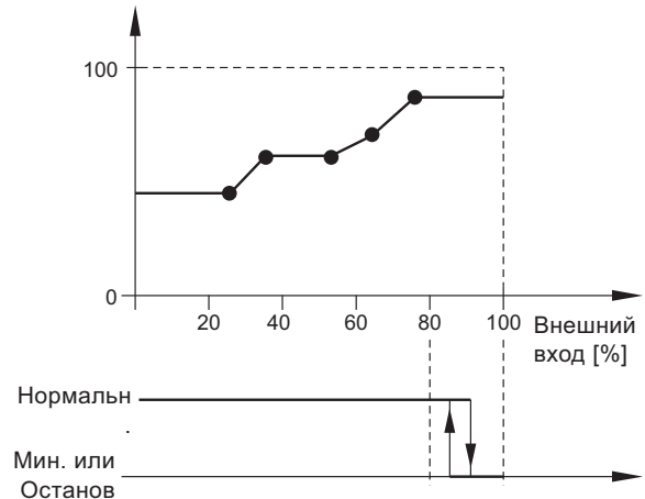
Рис. 49 Таблица влиян. с остан. у макс.
