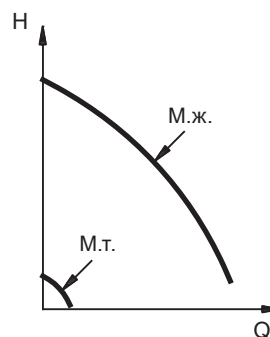
14-сур. Минималды және максималды сипаттамалар
