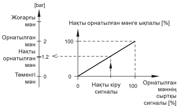
42-сур. Орнатылған мән реттеуін теңшеу мысалы
