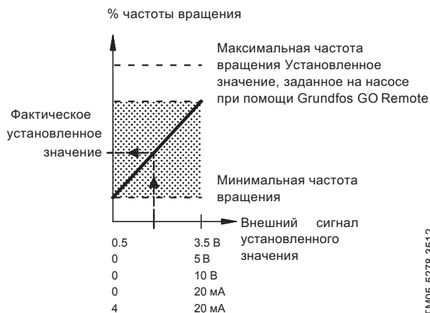
Рис. 25 Зависимость между фактическим установленным значением и внешним сигналом установленного значения при эксплуатации с постоянной характеристикой
