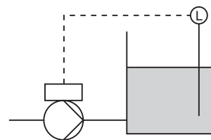
38-сур. Тұрақты деңгей
