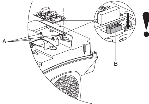
Рис. 60 Установка модуля SIM на одном уровне с пластиковыми держателями (поз. А) и подключение разъема (поз. В)
