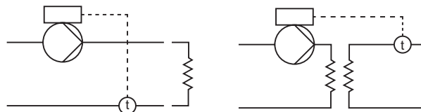
Рис. 30 Постоянная температура
