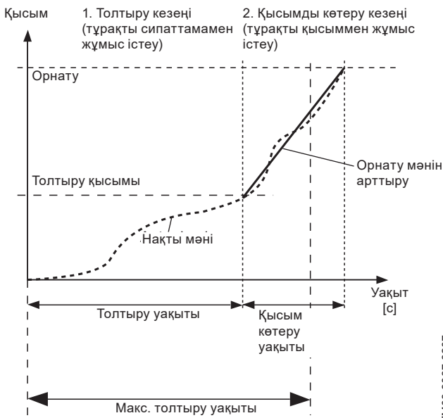
53-сур. Толтыру және қысым арттыру кезеңдері
