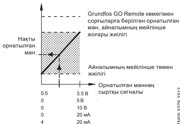
25-сур. Нақты орнатылған мән мен тұрақты сипаттама пайдалану кезіндегі орнатылған мәнің сыртқы сигналы арасындағы тәуелділік
