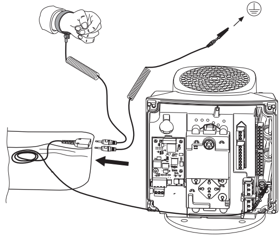
Рис. 56 Антистатический набор
