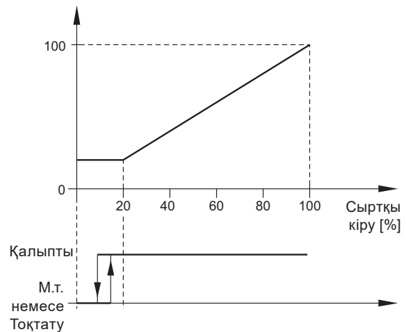
44-сур. «Тоқтатумен сызықтық» және «Мин сызықтық»
