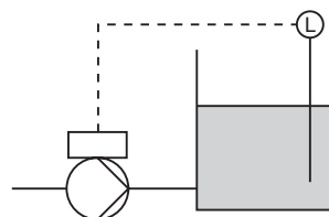
Рис. 38 Постоянный уровень
