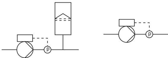
28-сур. Тұрақты қысым
