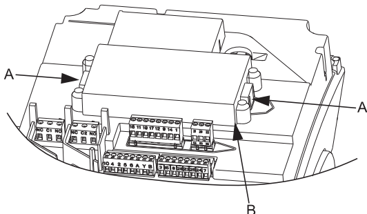
68-сур. Пластик қақпақты көтеру
