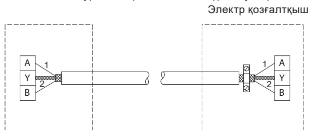
12-сур. 2 тарамды қоршалған кабельді қосу
