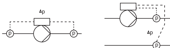
32-сур. Тұрақты қысым өзгерісі
