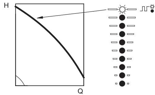
20-сур. Максималды сипаттама кезінде пайдалану
