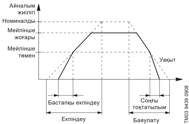
54-сур. Үдету және баяулату
