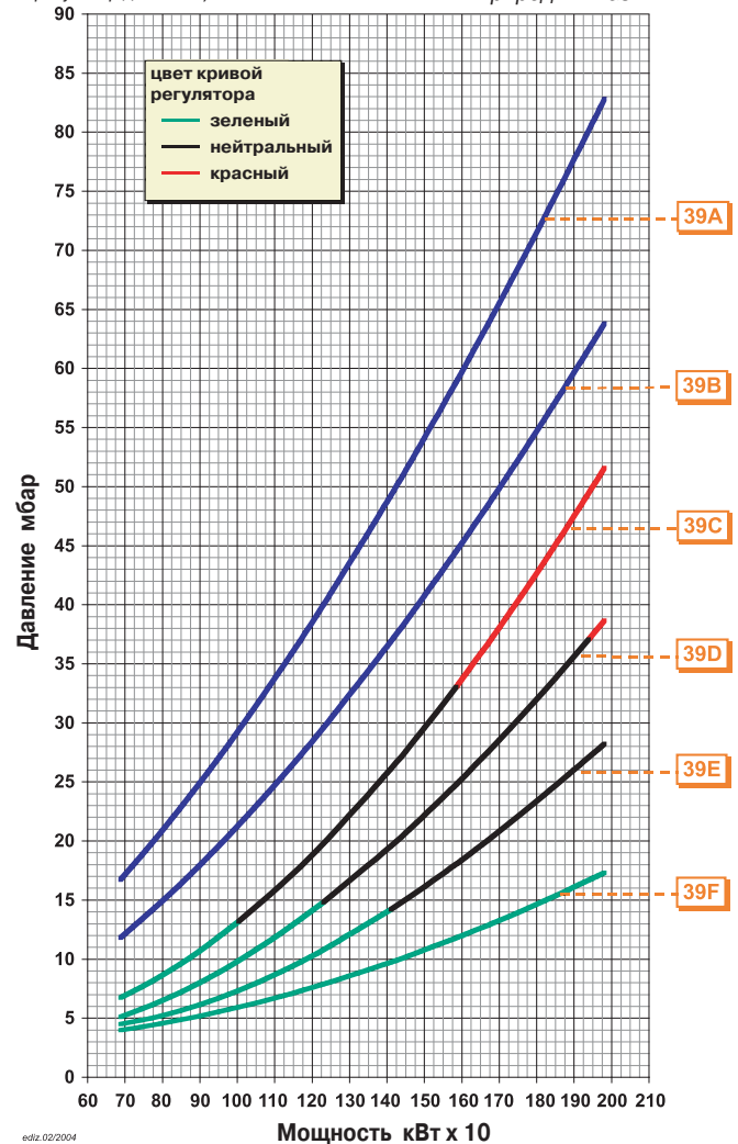
COMIST 180/180NM Природный газ
