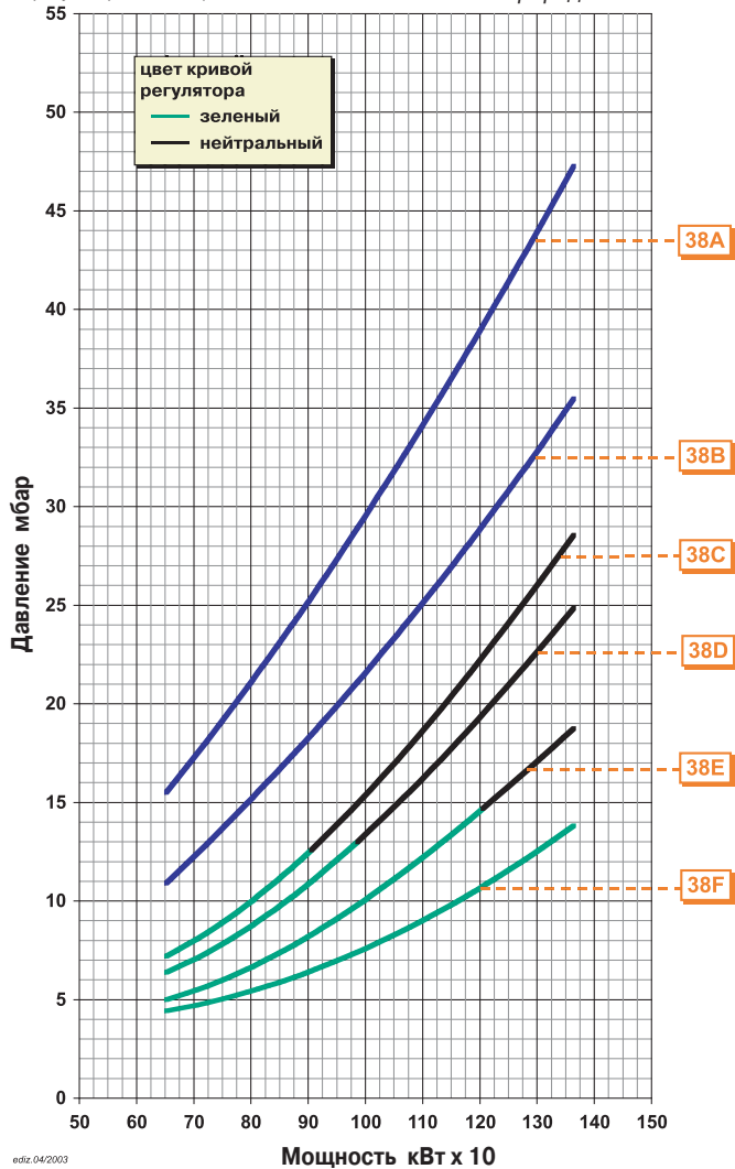
COMIST 122/122N Природный газ
