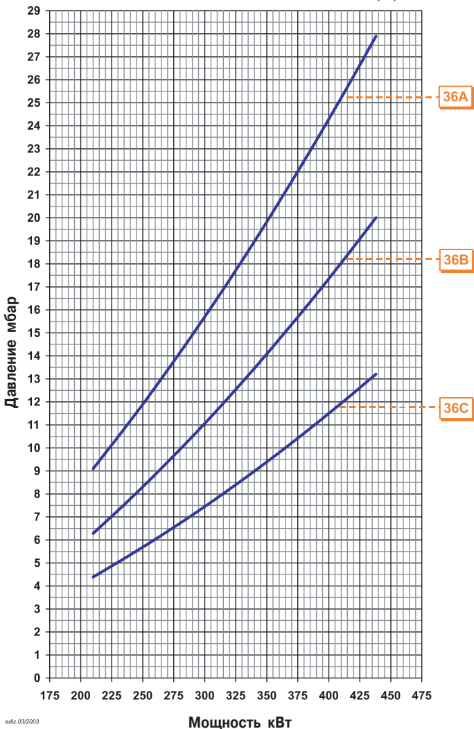
COMIST 36 Природный газ
