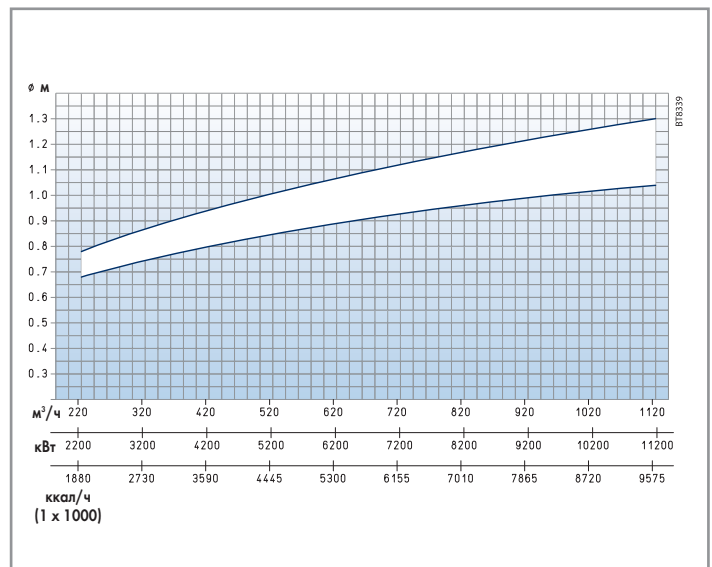
Зависимость диаметра пламени от количества сгоревшего газообразного топлива (приблизительные величины)
