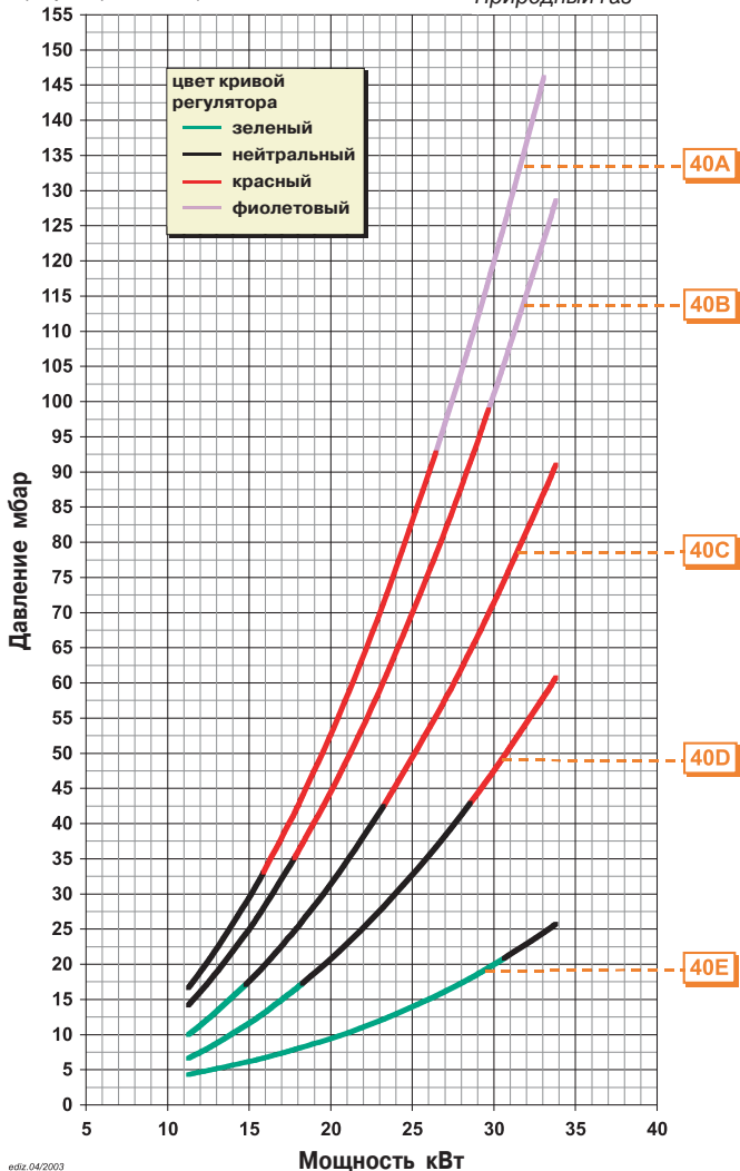
COMIST 250/250NM Природный газ
