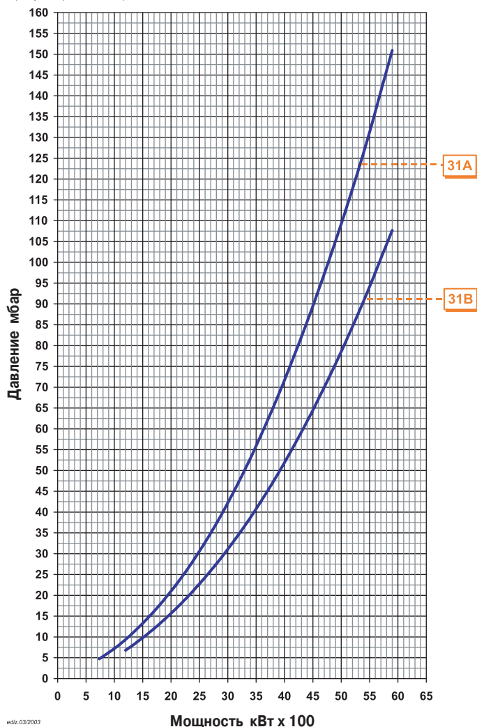
BGN 540LX Природный газ
