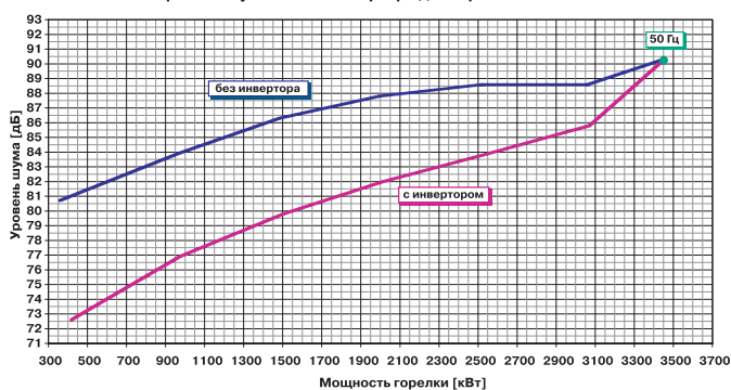
Уровень шума с и без инвертера для горелок BGN 300LX
