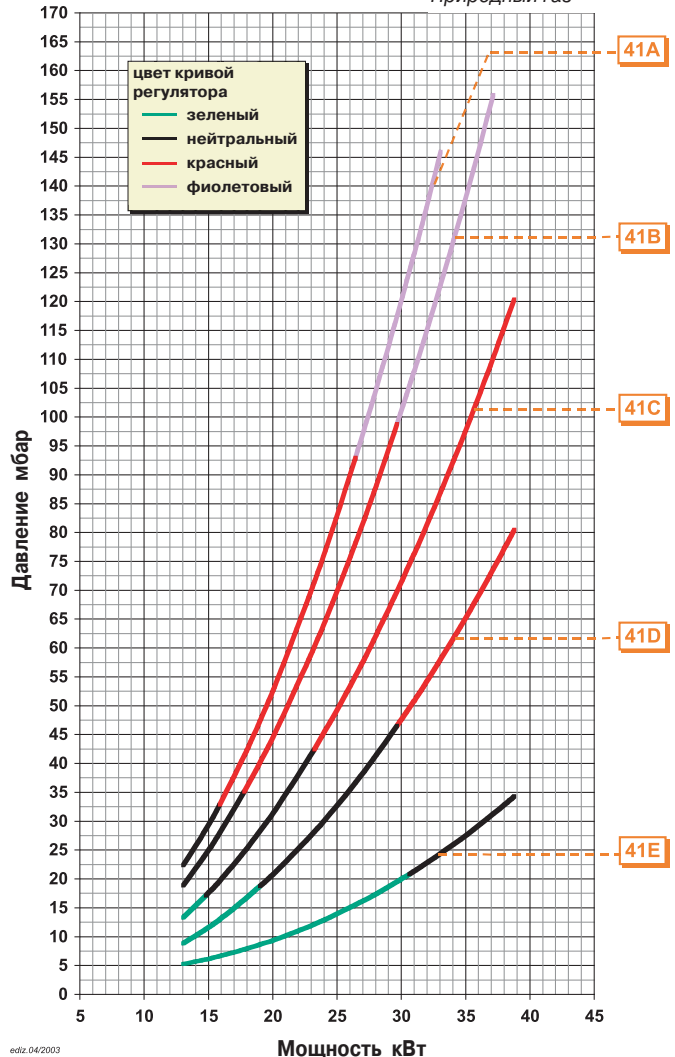
COMIST 300/300NM Природный газ
