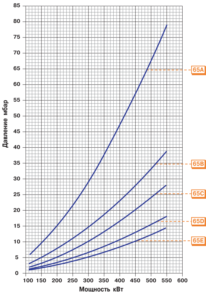
ТВГ 55 Р Природный газ
