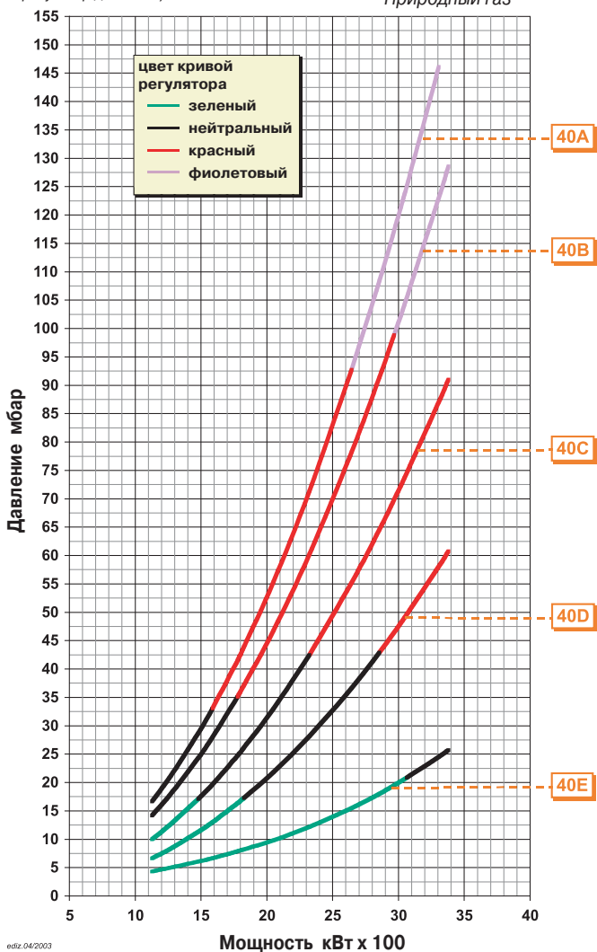
COMIST 250/250NM Природный газ
