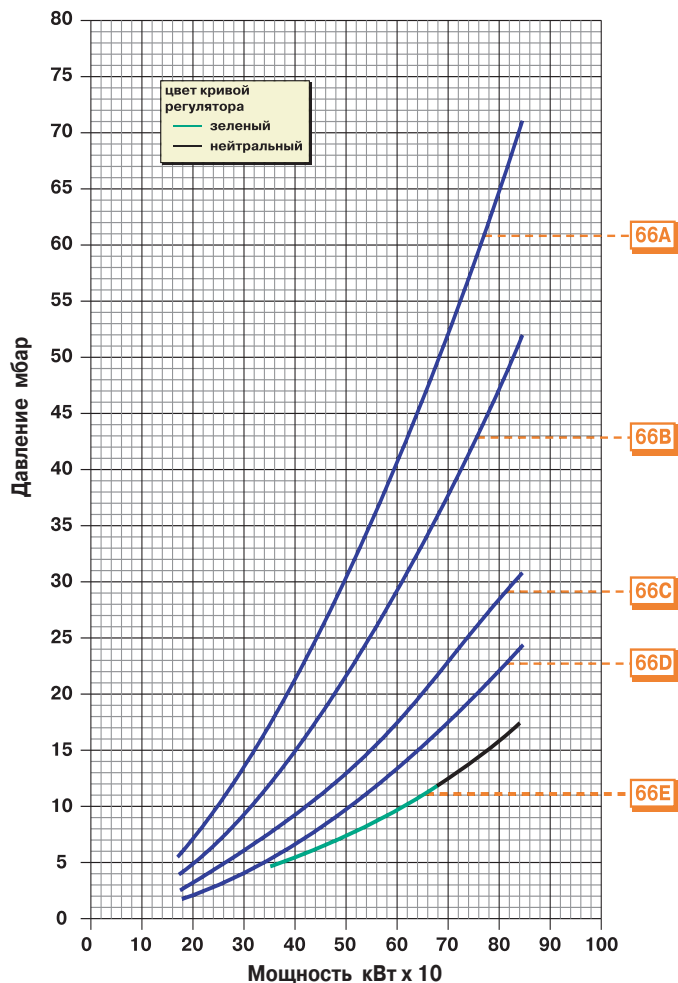
ТВГ 85 Р Природный газ
