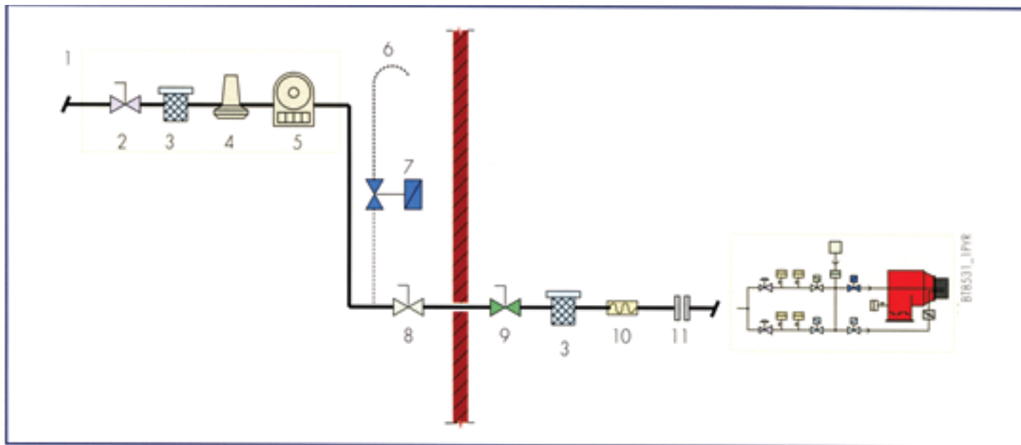
Принципиальная схема подсоединения горелки к газовой сети среднего давления
