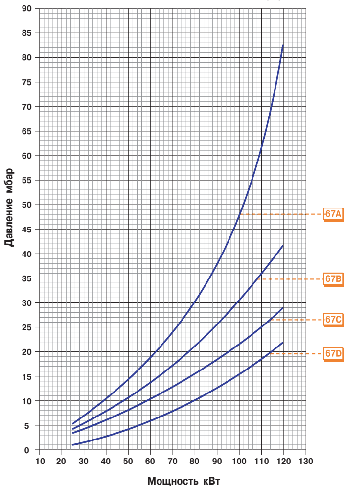
TBG 120PN Природный газ
