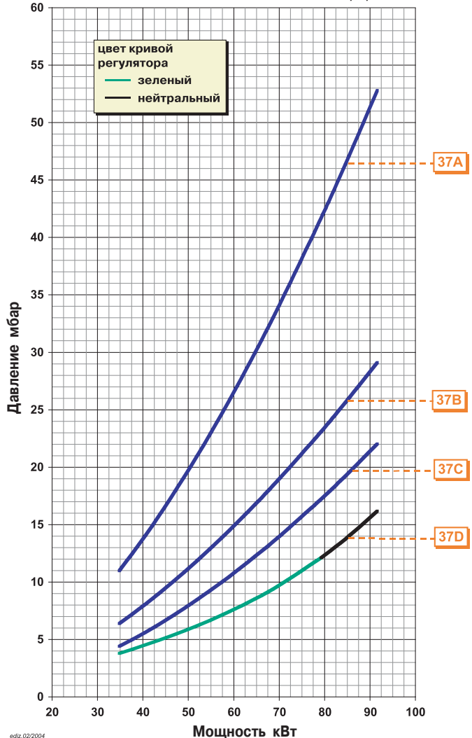
COMIST 72/72N Природный газ
