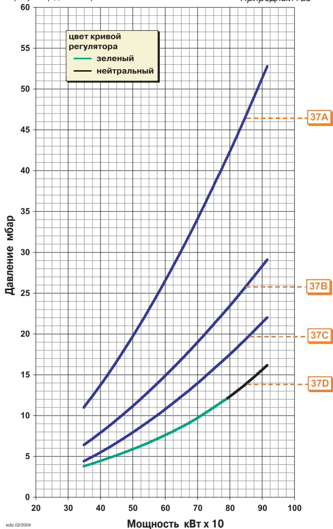
Потери напора (сопловая сборка + газовая рампа + регулятор давления) COMIST 72/72N Природный газ
