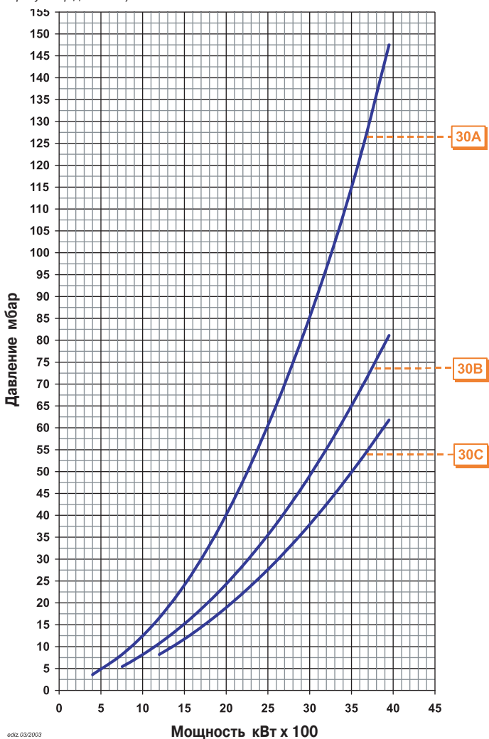
BGN 390LX Природный газ
