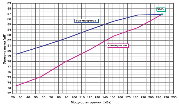
Уровень шума с и без инвертера для горелок BGN 200 LX
