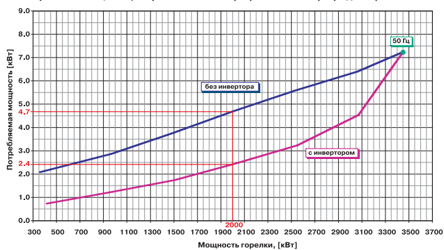
Электрическая мощность, потребляемая с инвертером и без инвертера для горелок BGN 300LX
