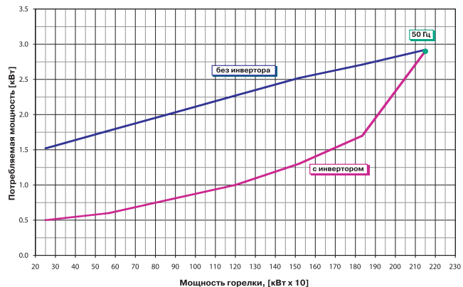
Электрическая мощность, потребляемая с инвертером и без инвертера для горелок BGN 200LX
