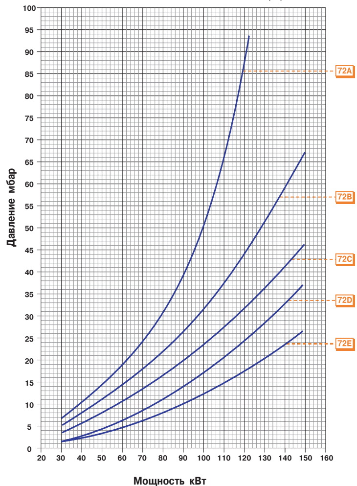
TBG 150PN Природный газ
