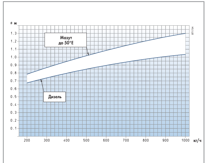
Зависимость диаметра пламени от количества сгоревшего мазута / дизельного топлива (приблизительные величины)
