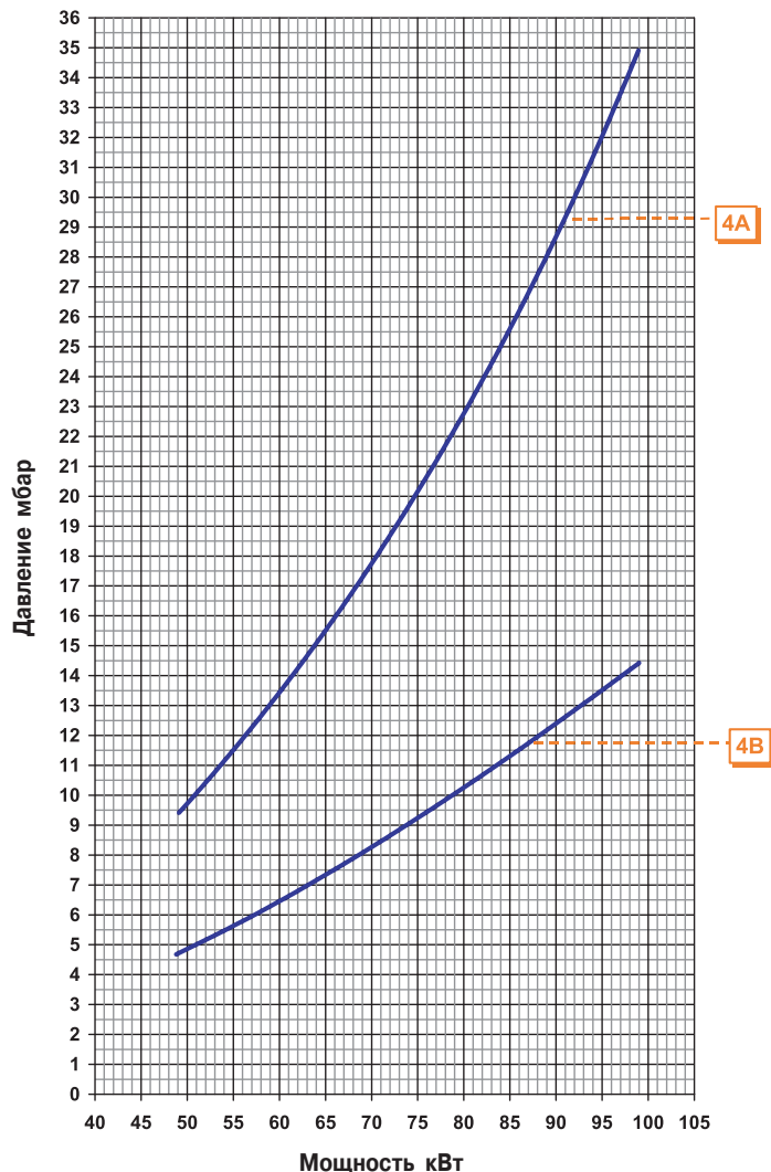
WSG 10 Природный газ
