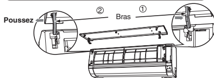
Retrait du panneau frontal
