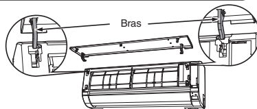
Fixation du panneau frontal
