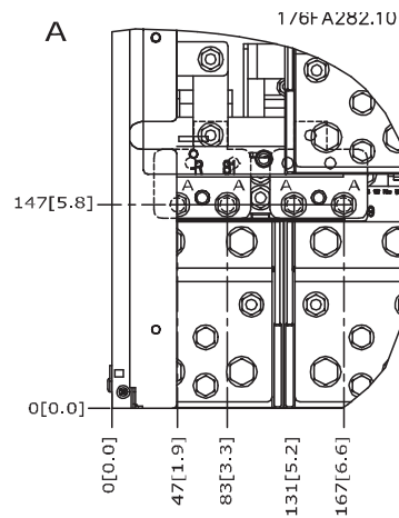
Рисунок 3.19: Расположение разъемов питания на корпусе IP00
