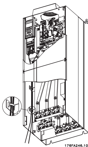
Схема подключения проводки платы управления D3. При подключении платы управления D1, D2, D4, E1 и E2 используется та же схема.
