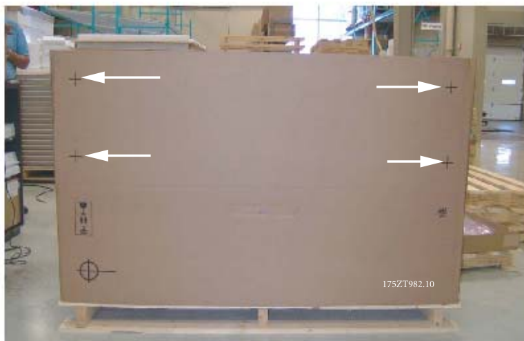
Рисунок 3.1: Монтажный шаблон
