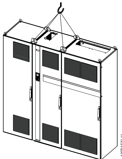
Рисунок 3.5: enclosure Рекомендуемый метод подъема, размер корпуса F3.
