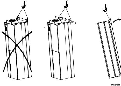
Рисунок 3.31: Способ подъема привода для монтажа на стене
