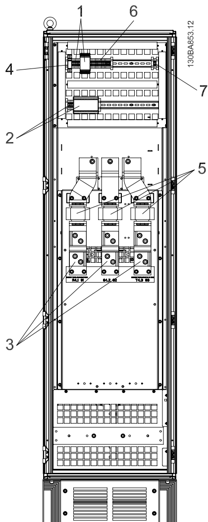
Рисунок 3.50: Дополнительный шкаф, размер корпуса F3 и F4
