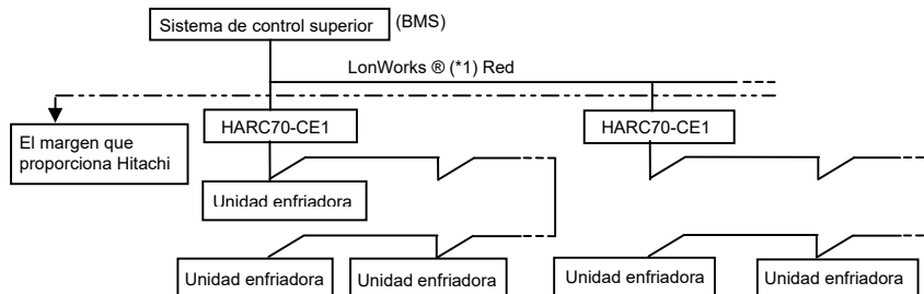
Fig. 1.1. Ejemplo de estructura del sistema
