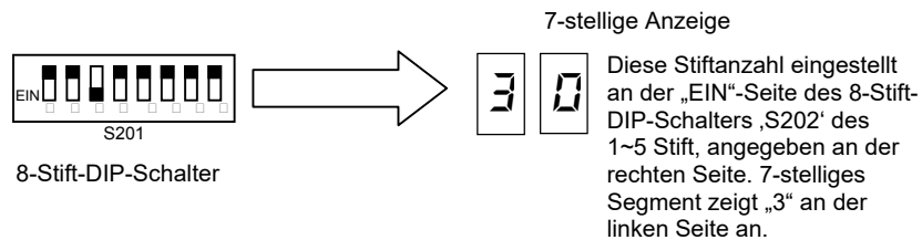
8-Stift-DIP-Schalter
