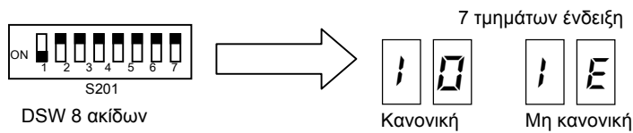
DSW 8 ακίδων
