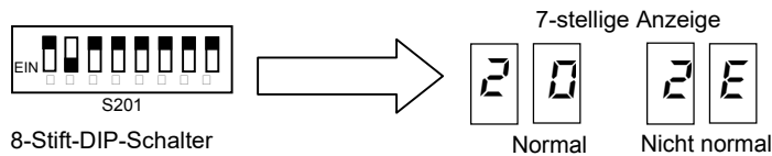
8-Stift-DIP-Schalter
