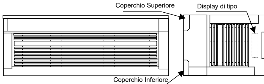
Fig. 1.3. Aspetto esterno di HARC70-CE1
