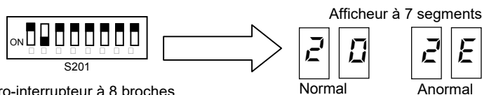
Micro-interrupteur à 8 broches
