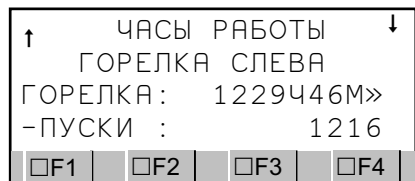
Изобр. 27: Часы работы левой горелки котла с двумя жаровыми трубами
