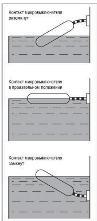
Рис. 3. Принцип действия поплавкового выключателя
