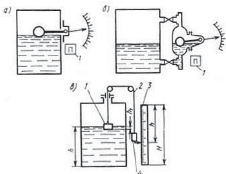
Рис. 2. Схемы поплавковых уровнемеров
