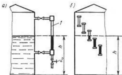
Рис. 1. Уровнемерные стекла
