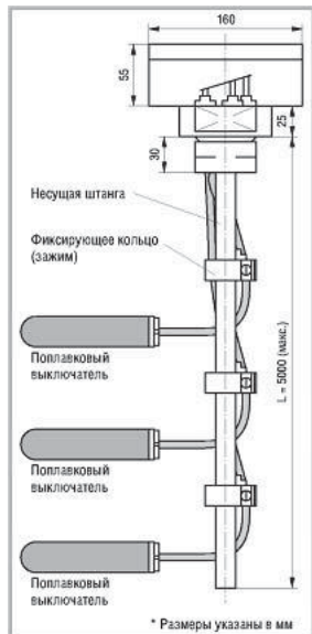
Рис. 5. Регулируемое устройство.
