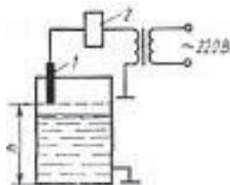
Рис. 17. Уровнемер кондуктометрический
