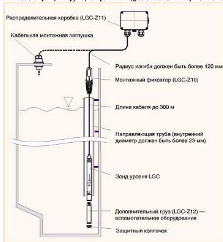
Рис. 11. Пример установки гидроstaticкого зонда уровня
