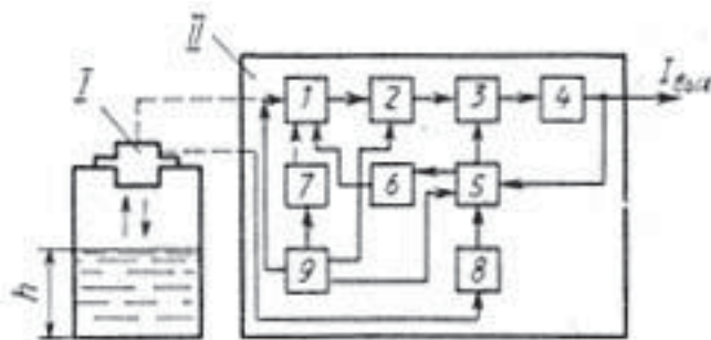
Рис. 20. Схема акустического уровнемера.
