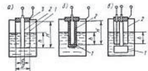
Рис. 14. Ёмкостные уровнемеры.
