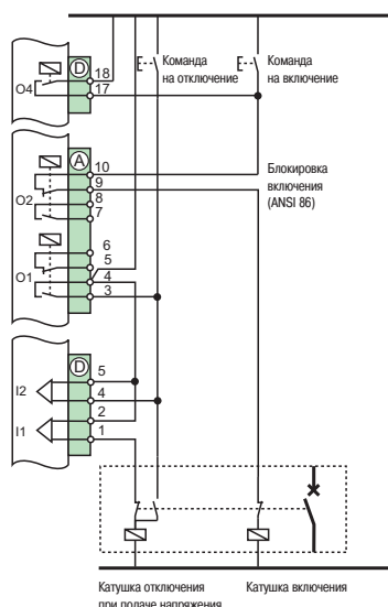
Управление выключателем с помощью Serwat серии 10 A
