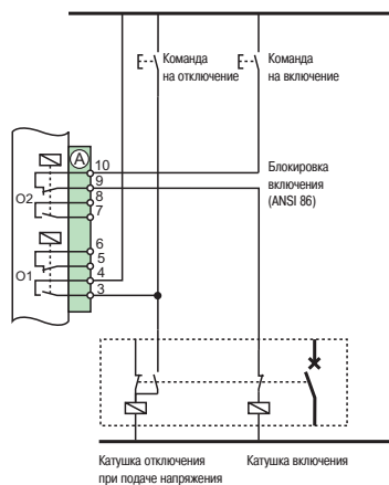
Управление выключателем с помощью Serwat серии 10 B
