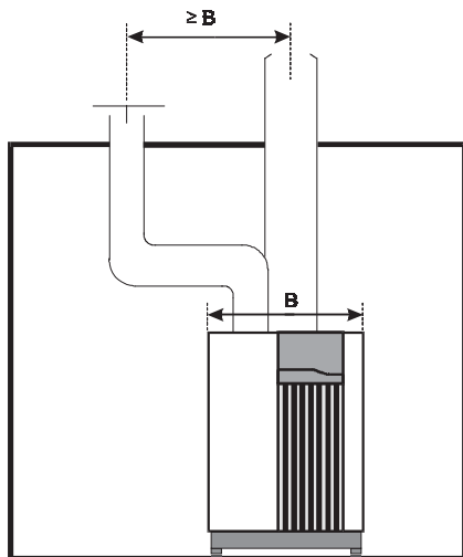
Рис. 21 Расстояние между входом воздуховода и выходом дымохода
