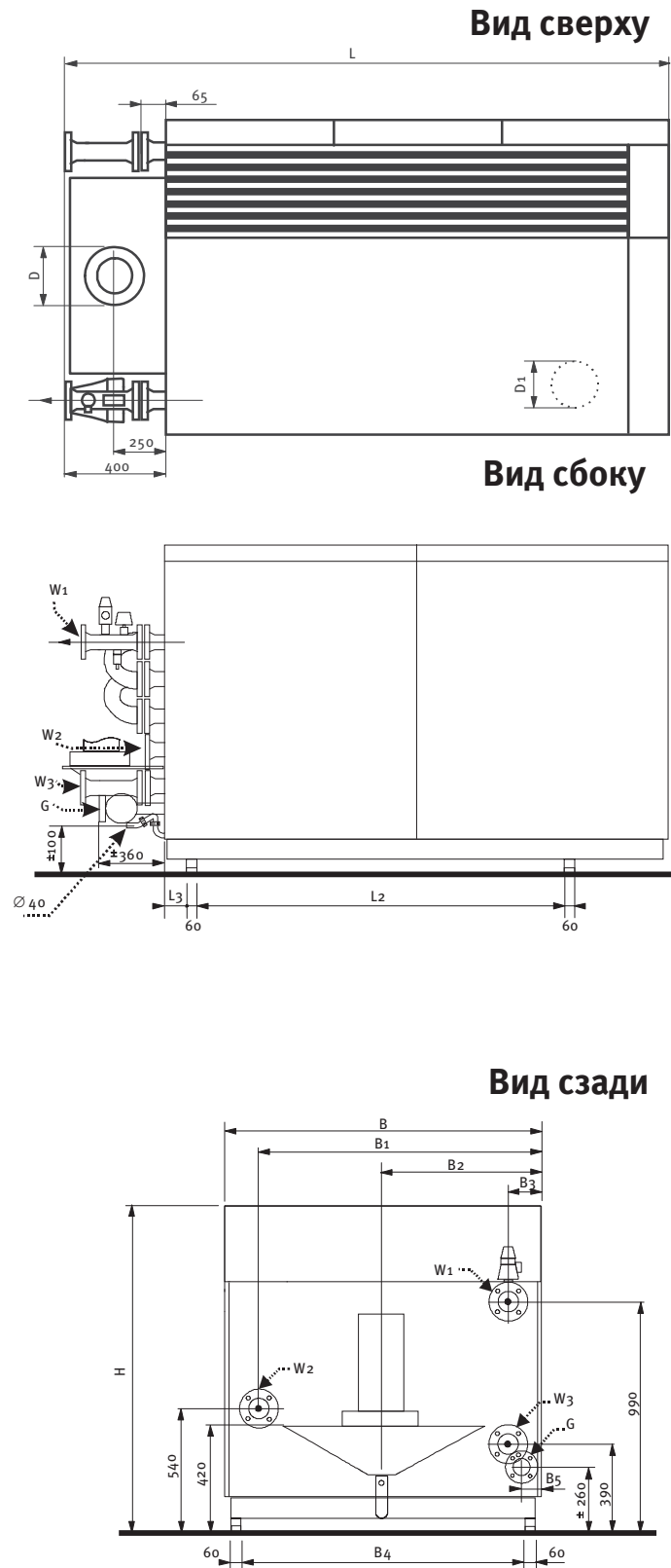
Рис. 34 Габариты R3600SB с раздельной системой.
