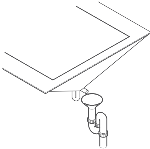
Рис. 23 Отвод конденсата
