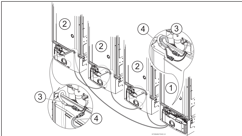
Rys. 2 Przykładowy montaż
