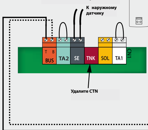
Схема водонагревателя
