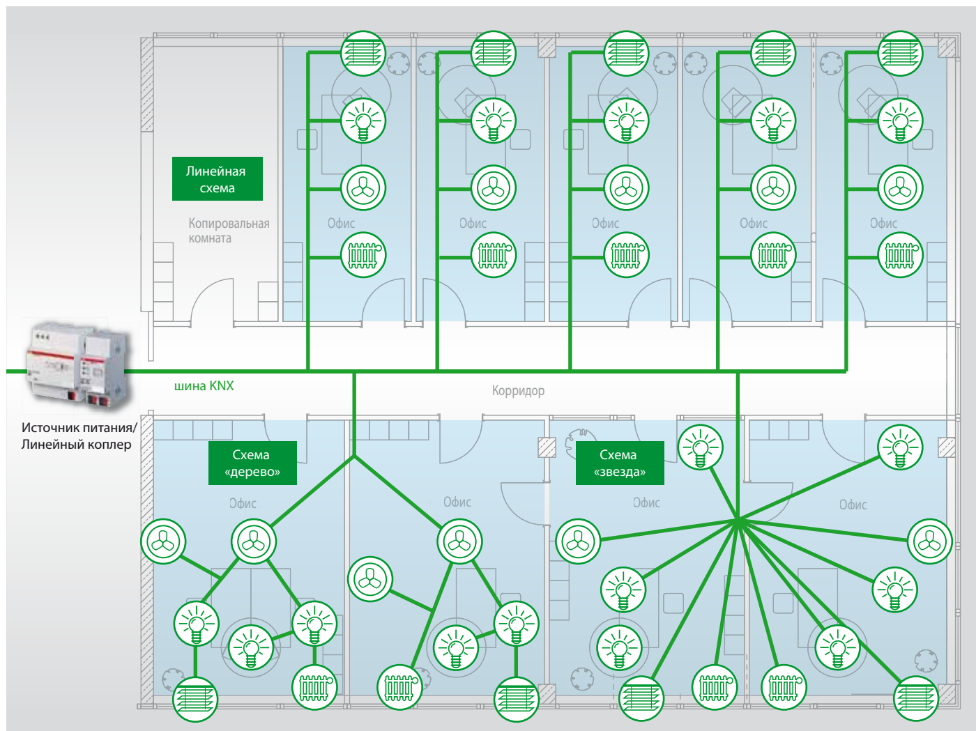
Схематическое представление шины KNX
